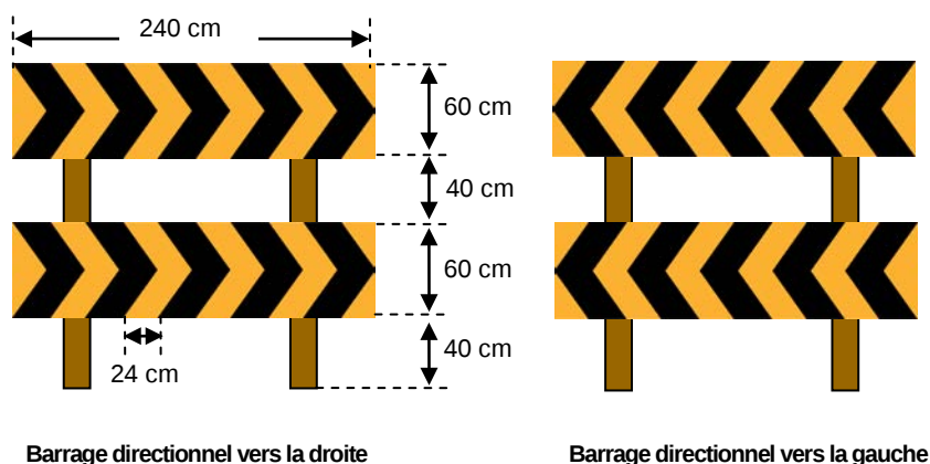
Figure 3-3 : Barrages directionnels
